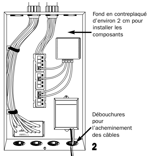
Système type de transmission de la voix/de données
